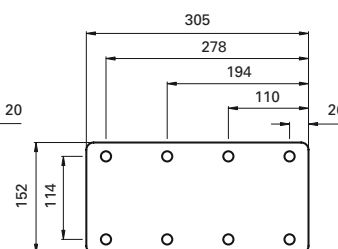
TRAD. BASEPLATE 200, 225, 250
