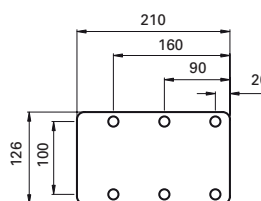
TRAD. BASEPLATE 100, 125, 150, 175
