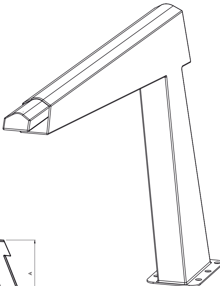
TRAD. BASEPLATE 100, 125, 150, 175
