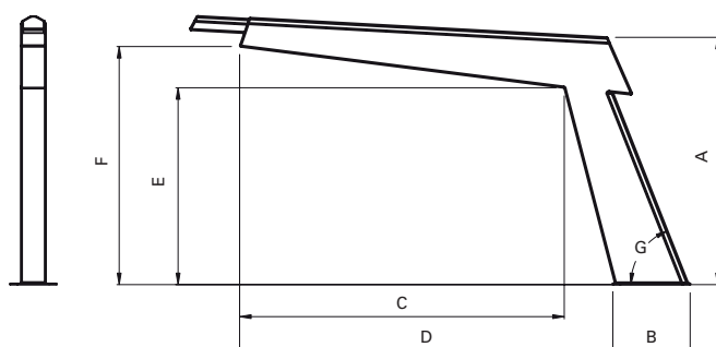
TRAD. BASEPLATE 100, 125, 150, 175
